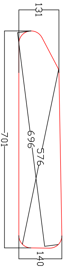
Måttene anger Hål i båt
