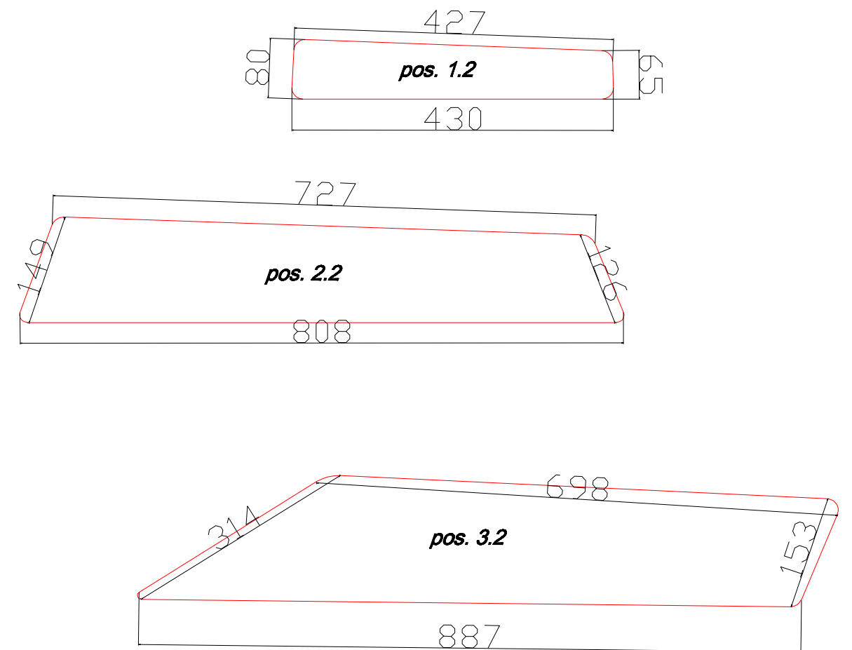
Mått hål i båt
